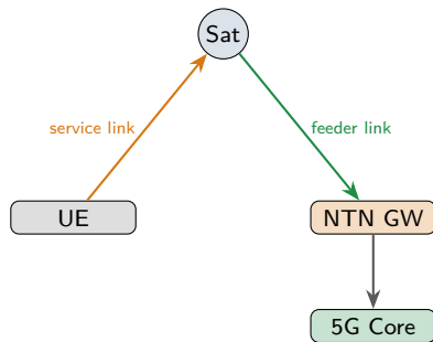
Figura: UE \rightarrow satélite (service) \rightarrow gateway (feeder) \rightarrow 5G Core; payload transparente ou regenerativo.
