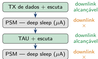
Figura: ciclo PSM no tempo: o UE só é alcançável nas janelas de escuta após acordar.
