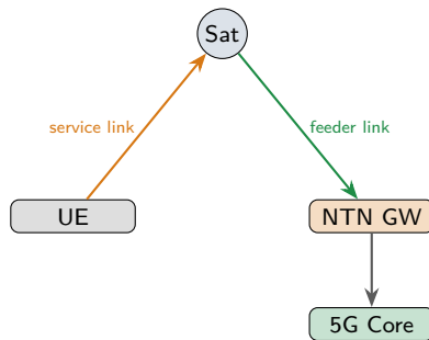
Figura 3: UE → satélite (service) → gateway (feeder) → 5G Core; payload transparente ou regenerativo.
