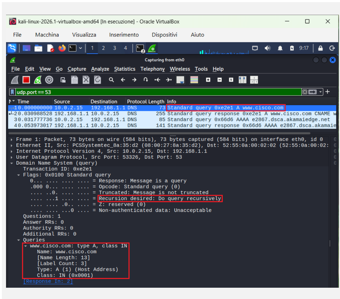
Figura 4 – Dettaglio della query DNS: Flags e sezione Queries espansa.
