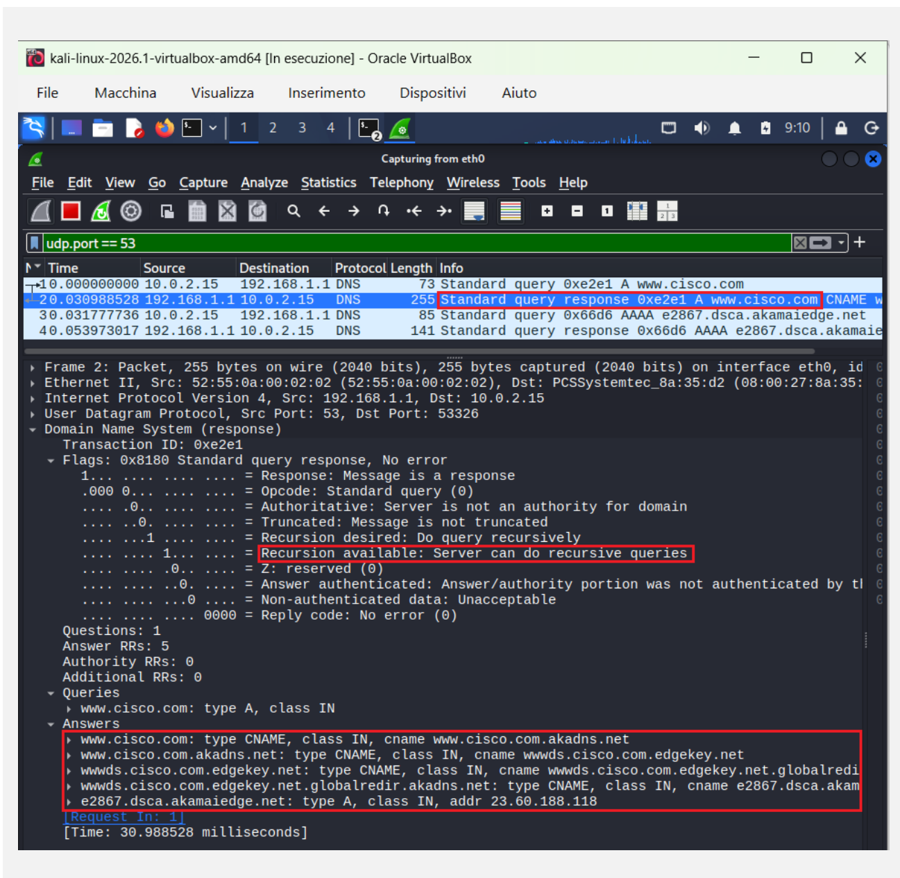
Figura 6 – Sezione Answers della risposta DNS: catena di record CNAME e record A finale.
