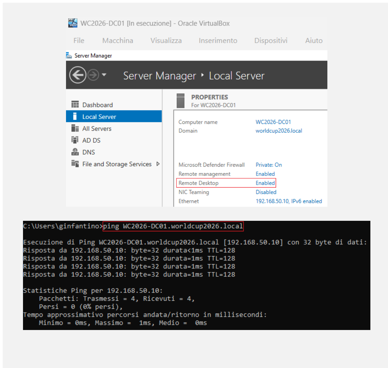
Figura 10 – Configurazione Remote Desktop e test di connettività ping verso WC2026-DC01
