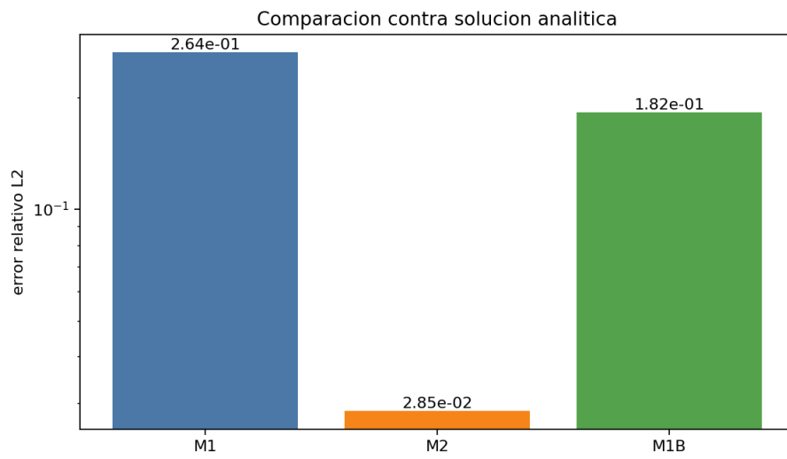
Figure 3: Ablacion extra: comparacion de M1, M1B y M2.
