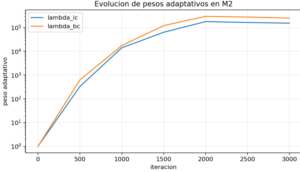
Figure 6: Evolucion de los pesos adaptativos de M2.
