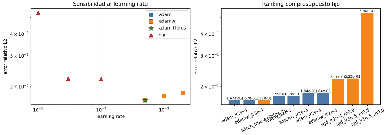
Figure 10: Comparacion de optimizadores con presupuesto fijo.
