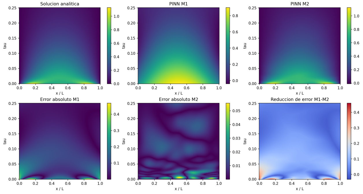
Figure 4: Solucion analitica, predicciones M1/M2 y mapas de error.
