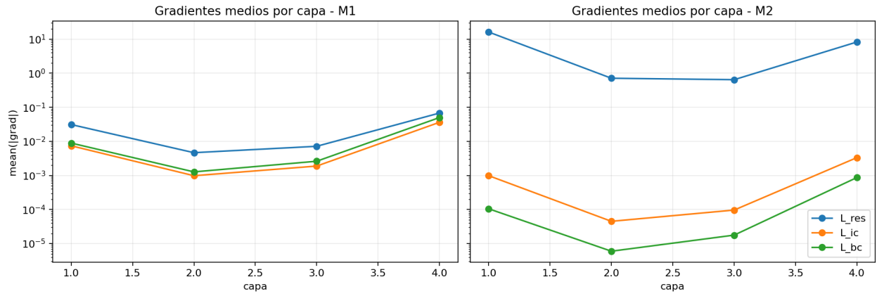
Figure 5: Diagnostico heredado del paper: magnitud media de gradientes por capa y por termino de perdida.
