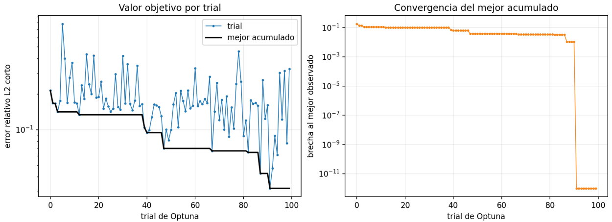
Figure 7: Historia de Optuna: objetivo por trial y mejor acumulado.
