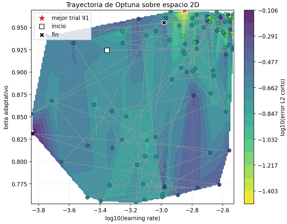
Figure 8: Trayectoria de búsqueda en el plano \log_{10}(\eta) - \beta .
