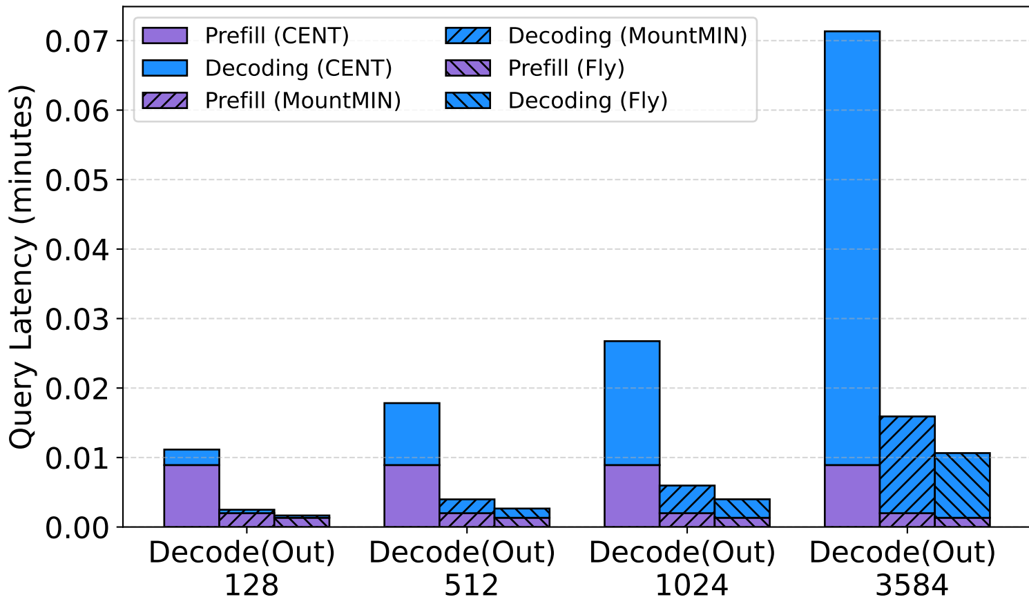
Llama2-70B - 32 Devices (Prefill-512)
