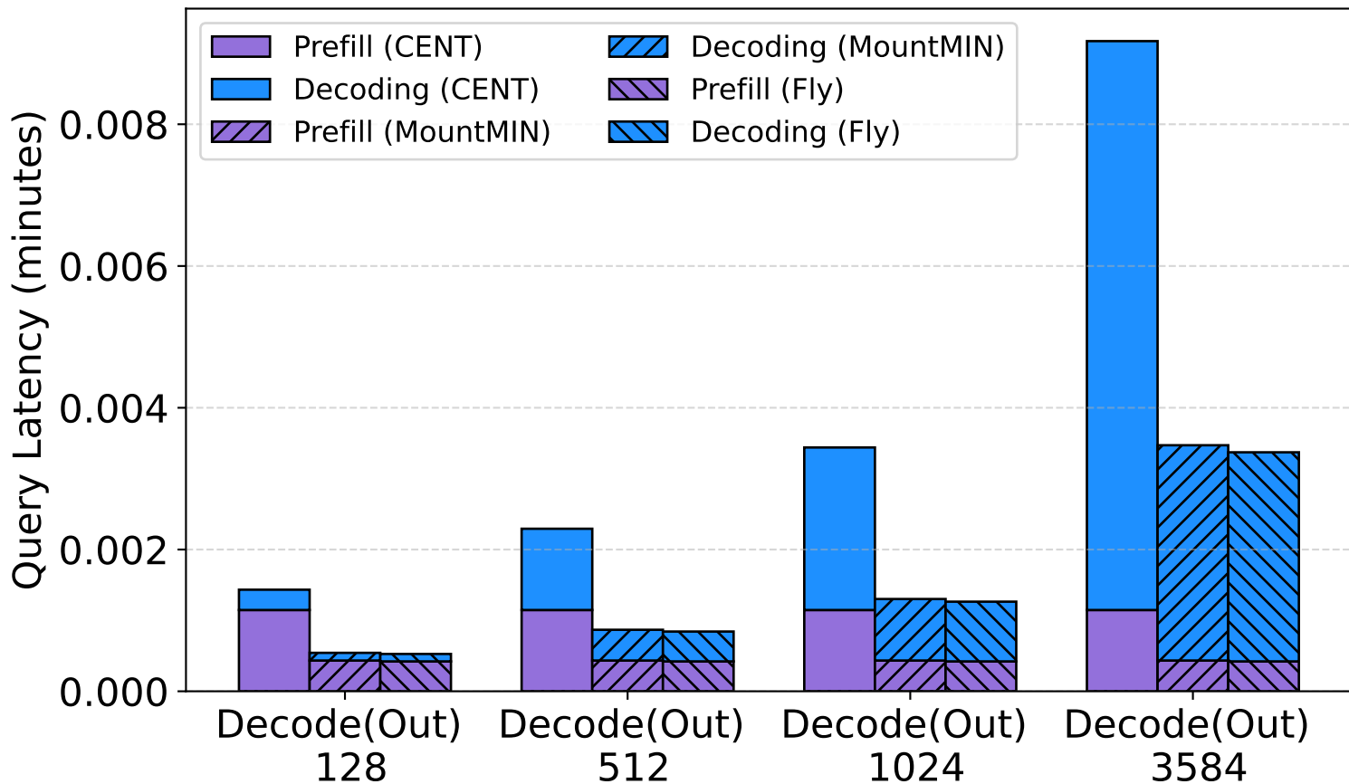
Llama2-7B - 32 Devices (Prefill-512)
