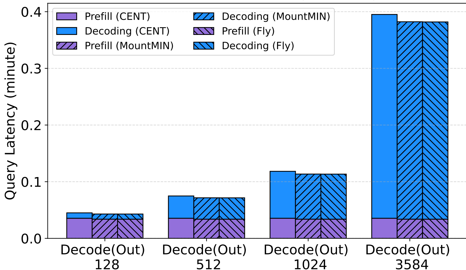
Llama2-7B - 20 Devices (Prefill-512)
