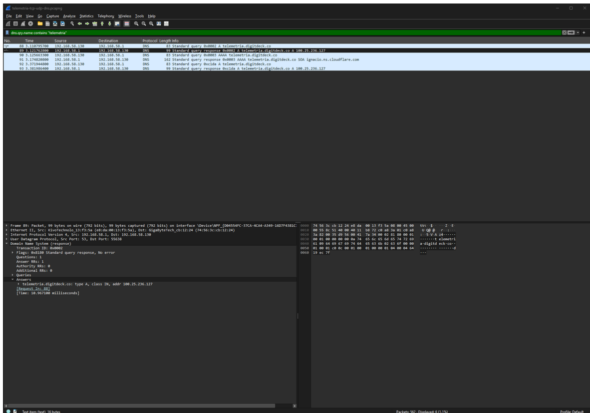
Figura 8. Wireshark con el filtro dns.qry.name contains "telemetria" : consulta A (paquete 88) al resolvedor 192.168.58.1 y respuesta (paquete 89) con 100.25.236.127 y TTL 260 s.
