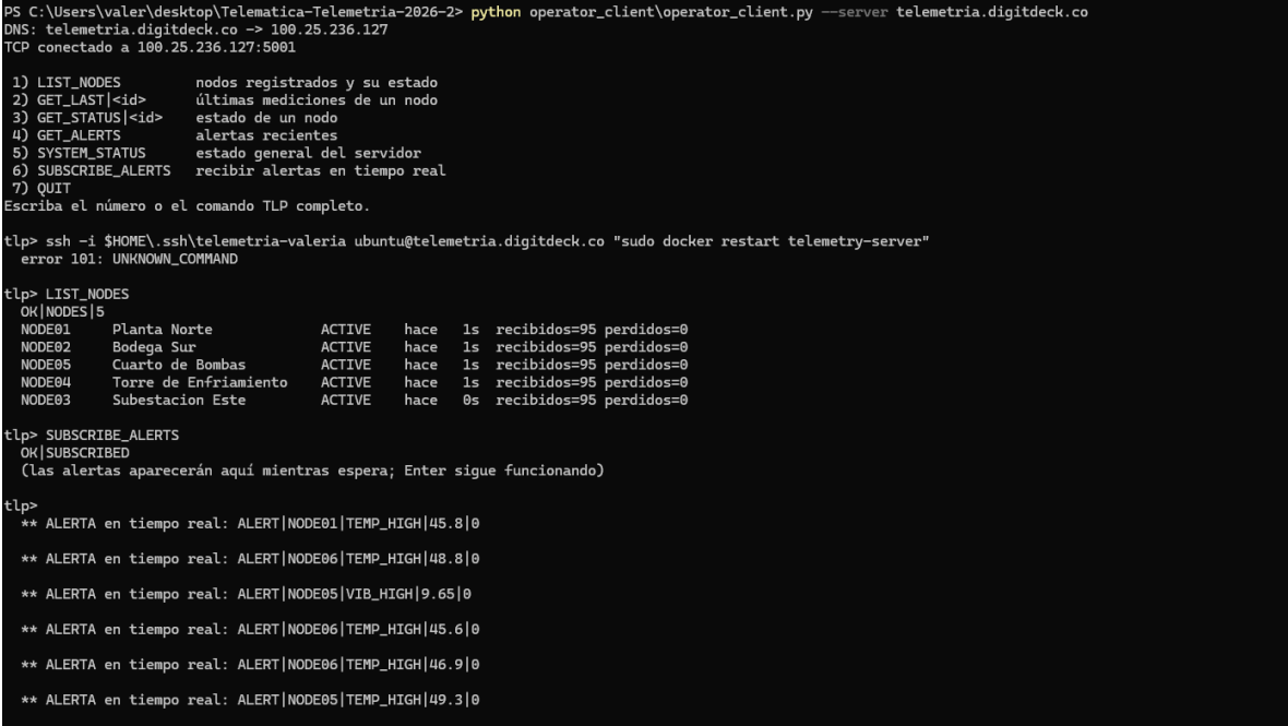
Figura 14. Cliente operador suscrito con SUBSCRIBE_ALERTS recibiendo alertas TEMP_HIGH en tiempo real desde un nodo con -force-alert TEMP.
