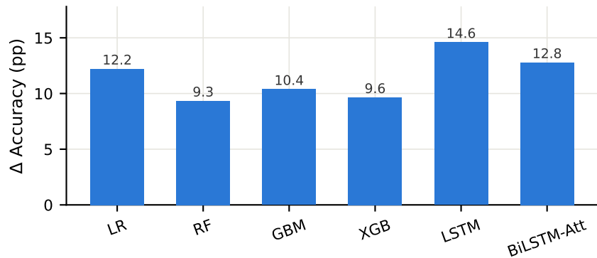
OULAD
