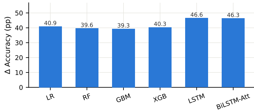
EdNet-KT1
