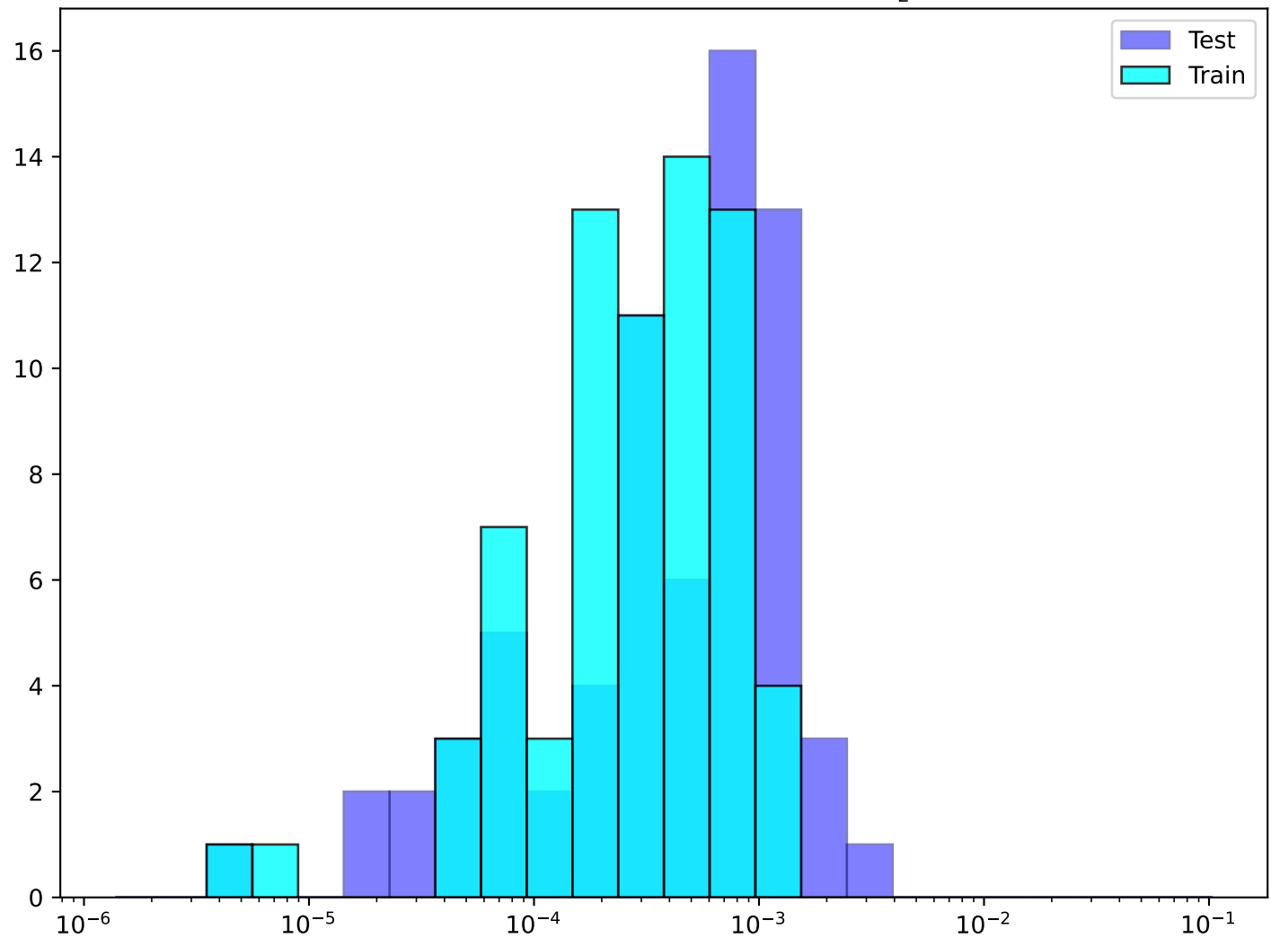
Distribution de l'Erreur Relative M_Z^2
