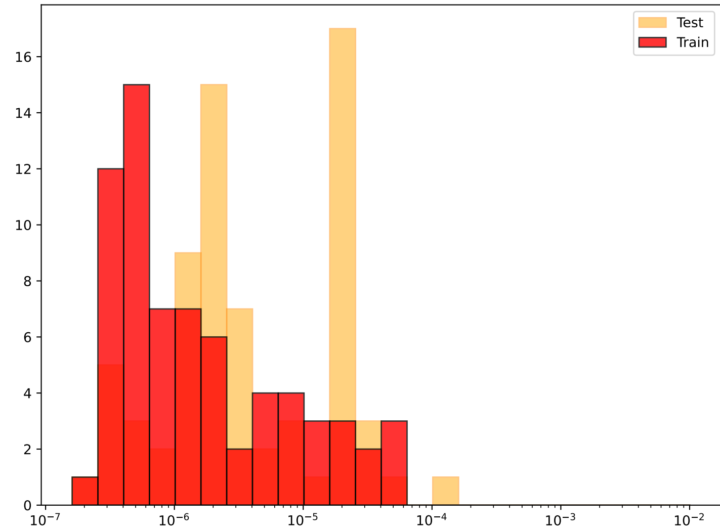
Distribution du V-score
