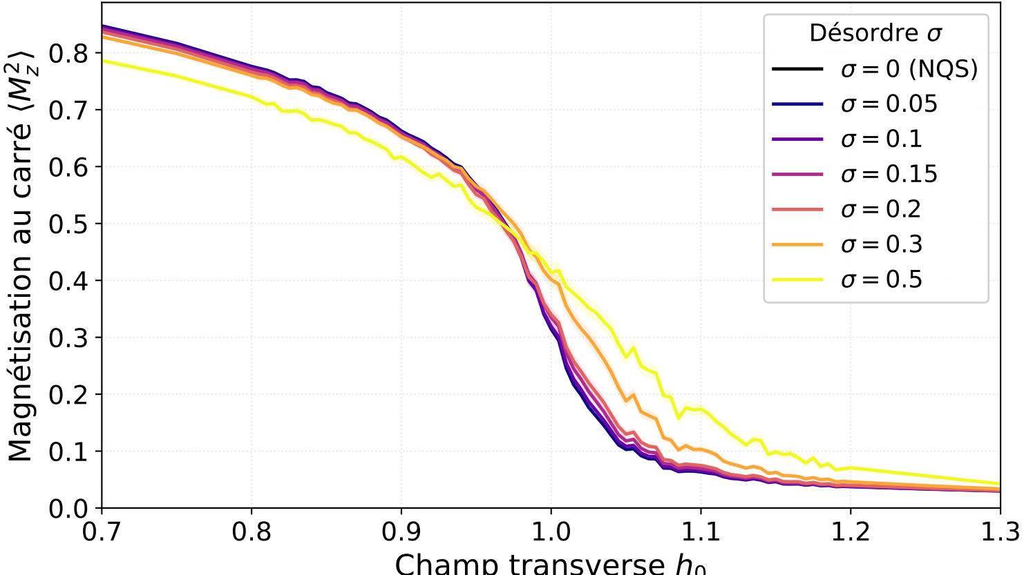
Chaîne d'Ising 1D, L = 120 spins (CLP)
