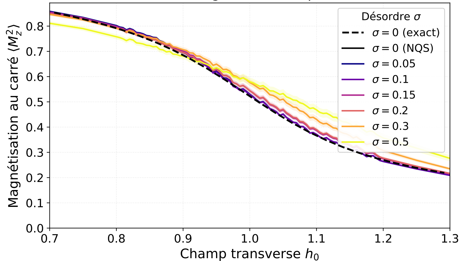
Chaîne d'Ising 1D, L = 16 spins (CLP)
