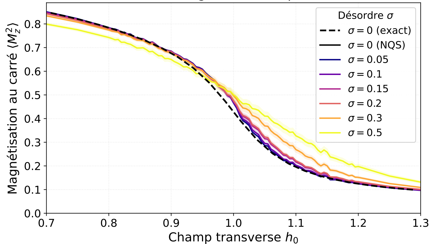
Chaîne d'Ising 1D, L = 36 spins (CLP)
