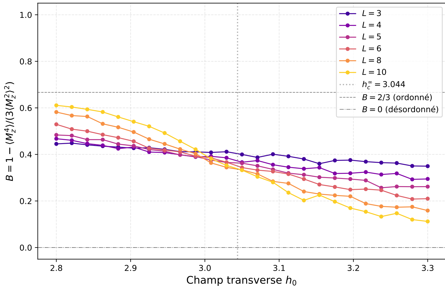
Binder cumulant — 2D TFIM sans désordre ( \sigma = 0 )
