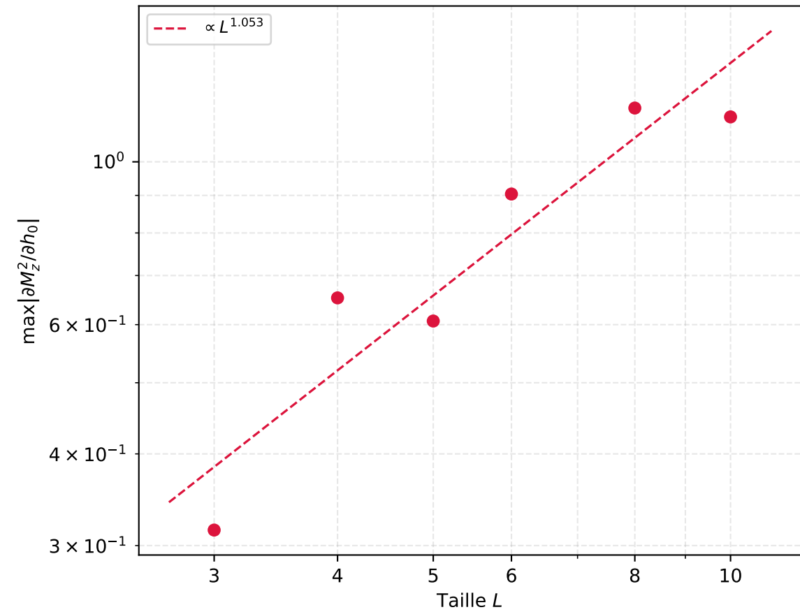
Pic de susceptibilité sans désordre vs L — \sigma = 0.0 (log-log)
