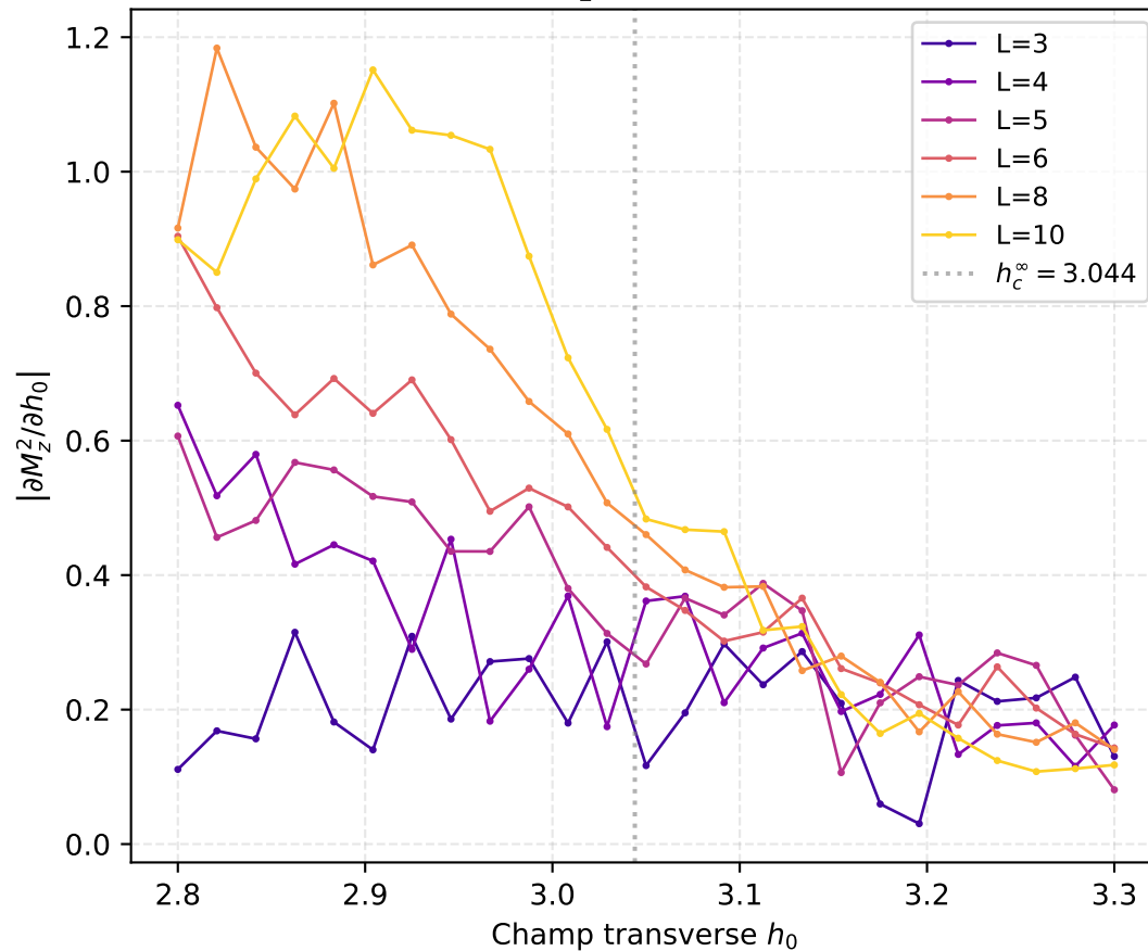
Dérivée de M_Z^2 (step=2) — \sigma = 0.0
