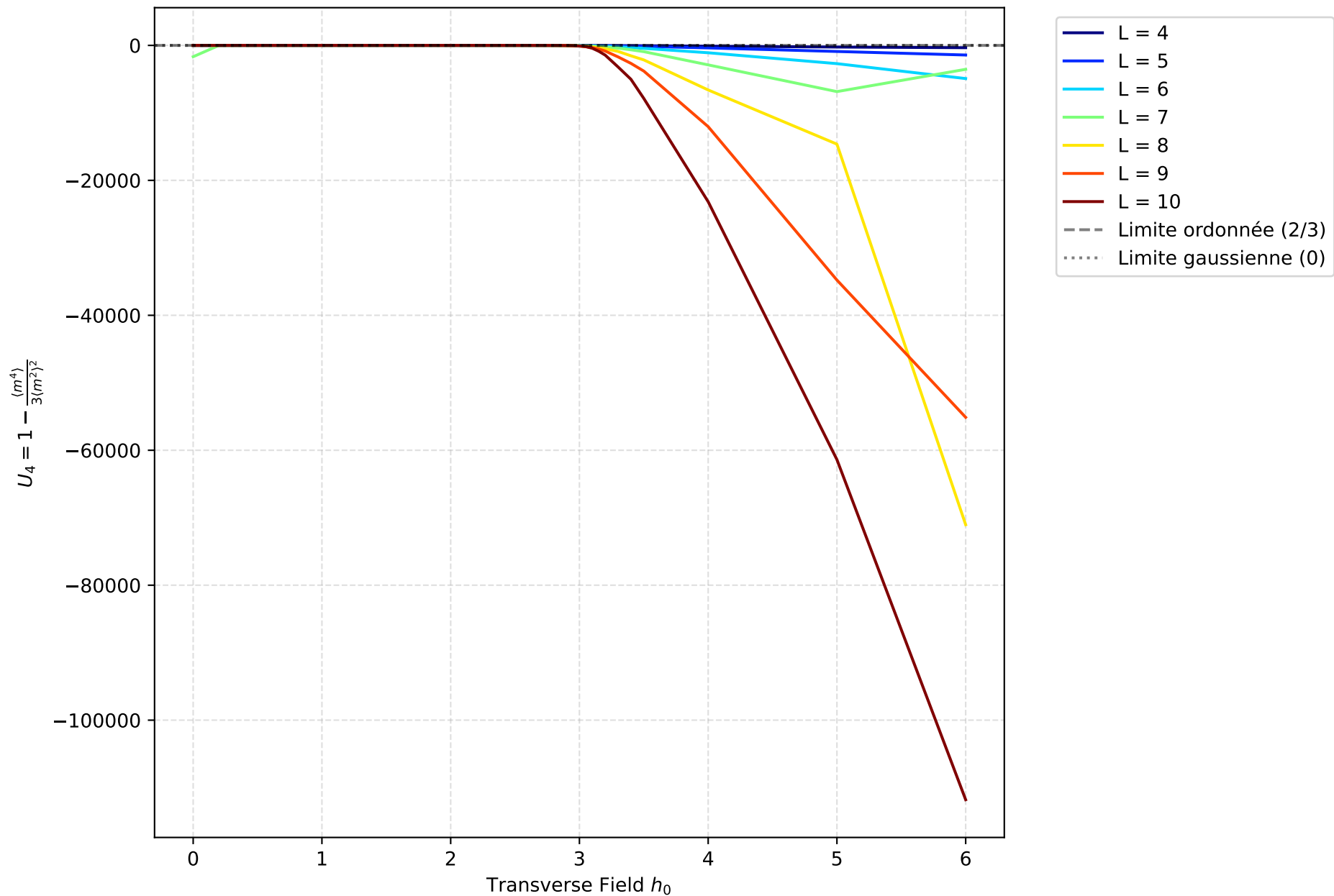
Binder Cumulant U_4 pour \sigma = 0.0 (2D System)
