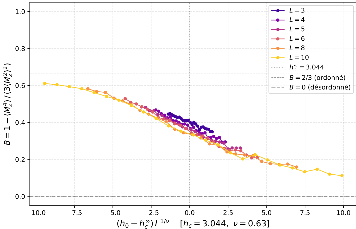
Binder cumulant collapsé — 2D TFIM sans désordre ( \sigma = 0 )
