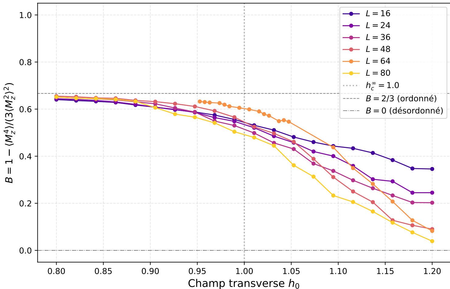
Binder cumulant — 1D TFIM sans désordre ( \sigma = 0 )
