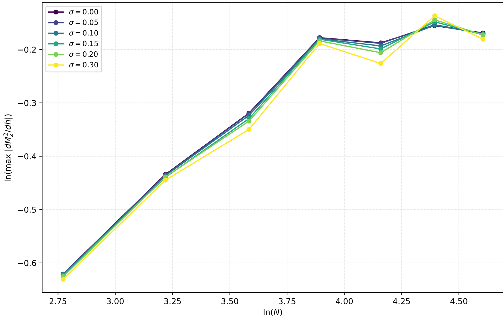
2D — Finite-Size Scaling par desordre
