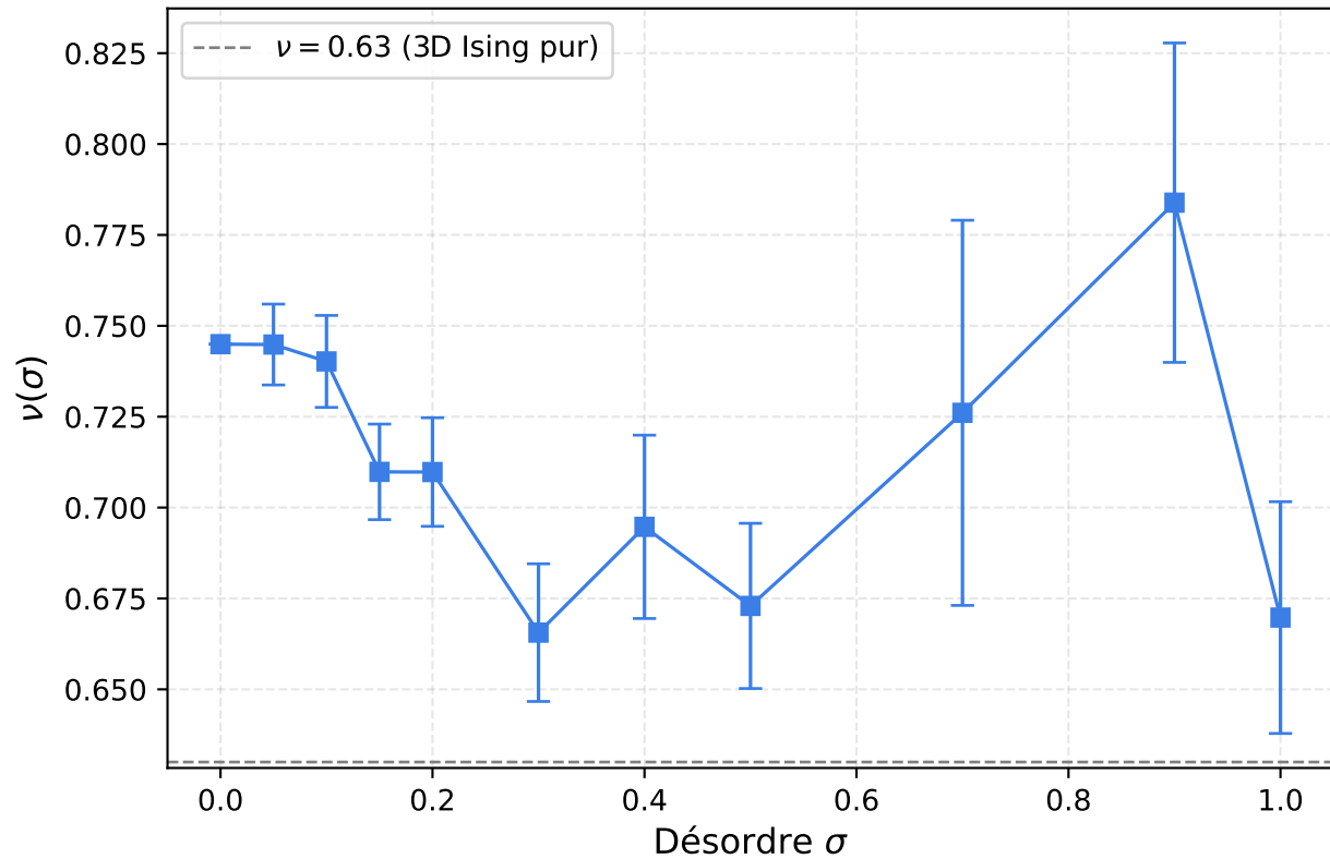
Exposant critique \nu vs désordre
