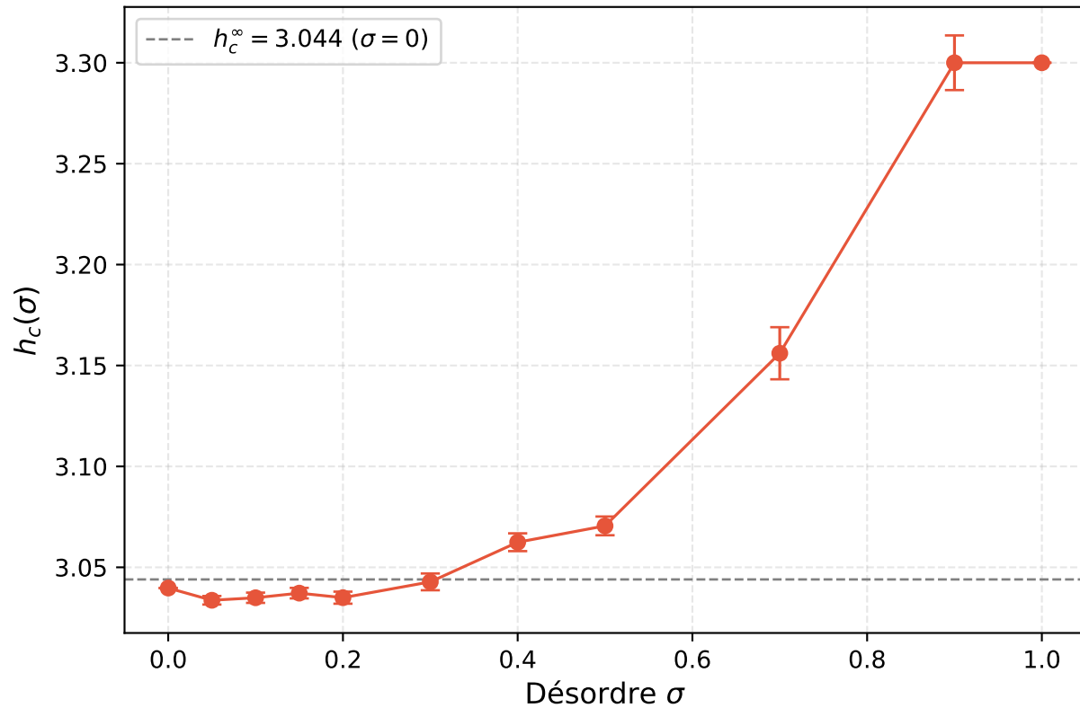
Point critique h_c vs désordre
