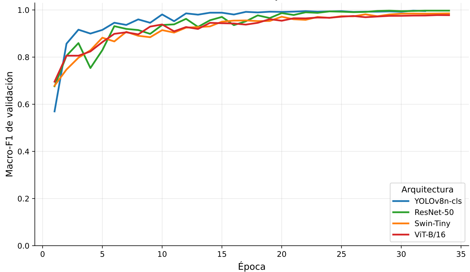
Macro-F1 de validación bajo CE balanceada
