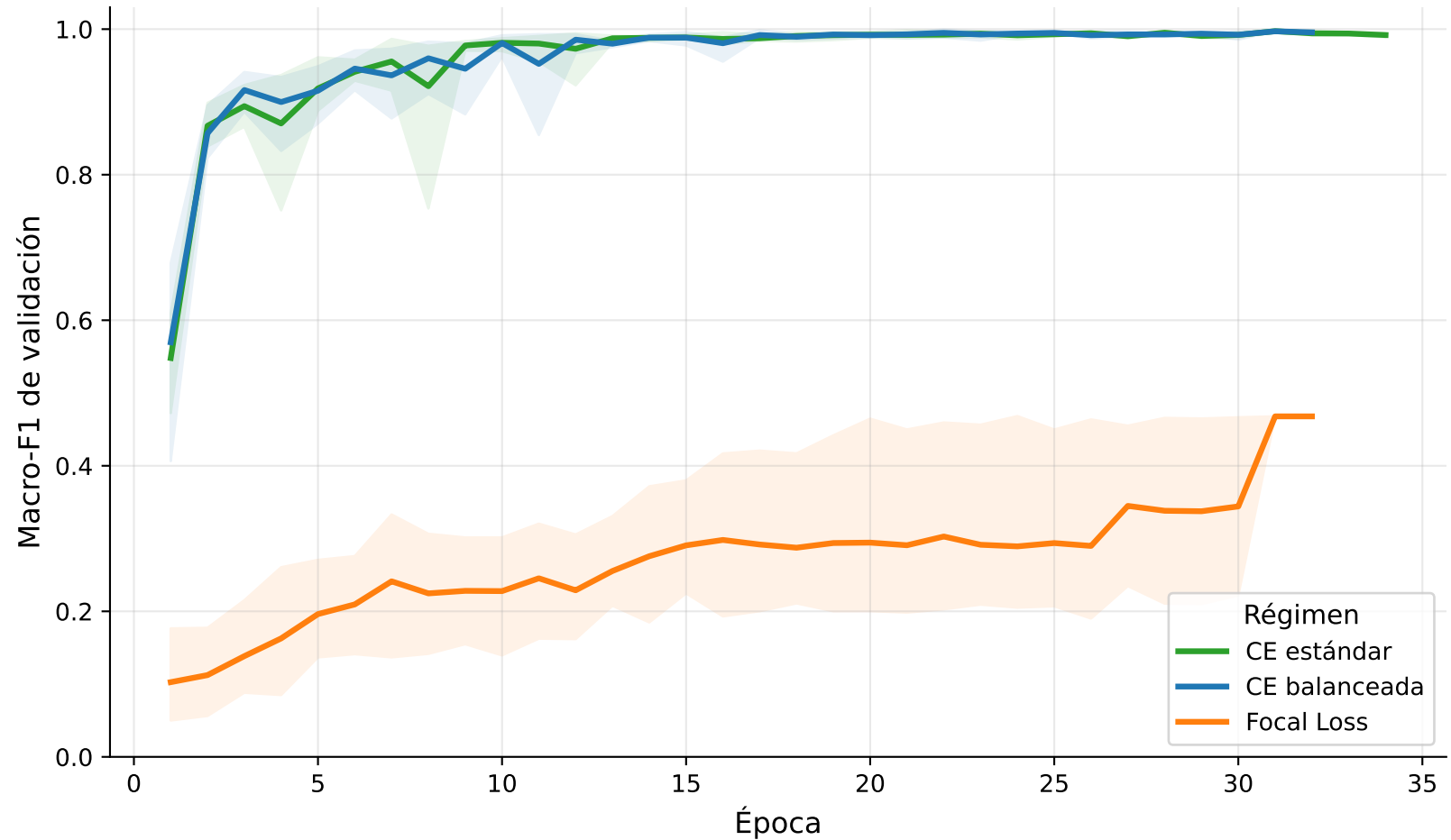
YOLOv8n-cls: Macro-F1 de validación por régimen
