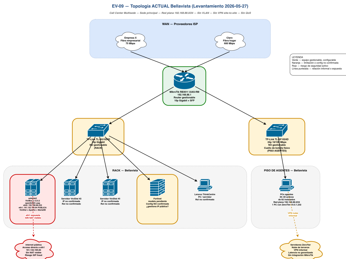
Figura 1: Topología lógica ACTUAL de la sede Bellavista — Red plana 192.168.88.0/24 sin segmentación VLAN, doble ISP sin failover y VPN informal ZeroTier preinstalada [8].
