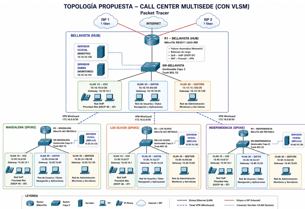
Figura 2: Topología lógica PROPUESTA del call center multisede — diseño basado en Hub-and-Spoke, segmentación de 3 VLANs por sede con VLSM, failover de ISP en Bellavista y VPN WireGuard centralizada [9].
