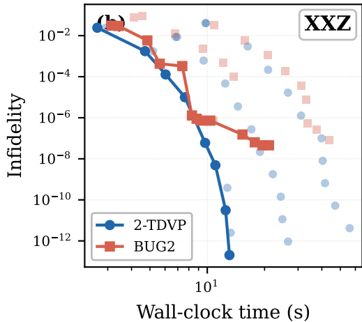
XXZ — Pareto frontier
