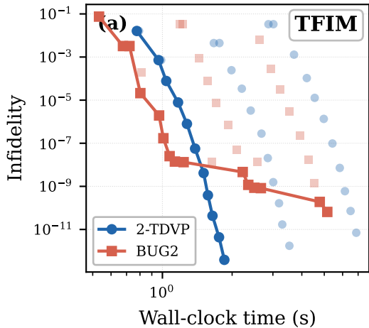
TFIM — Pareto frontier
