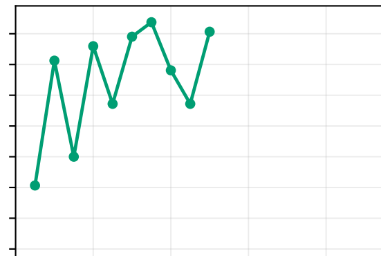
GRPO + DPO-Z
