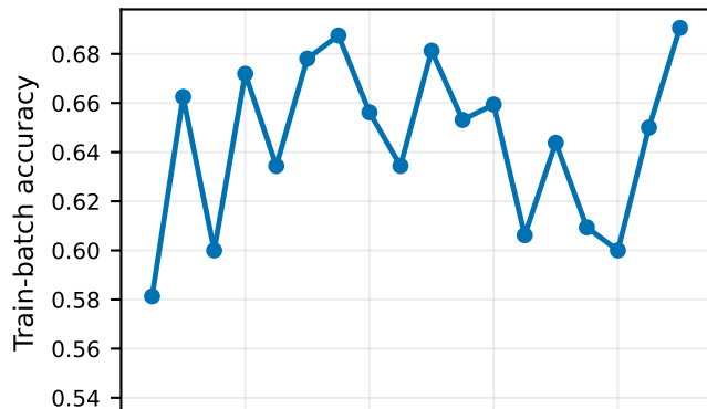
Vanilla GRPO
