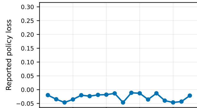
Vanilla GRPO
