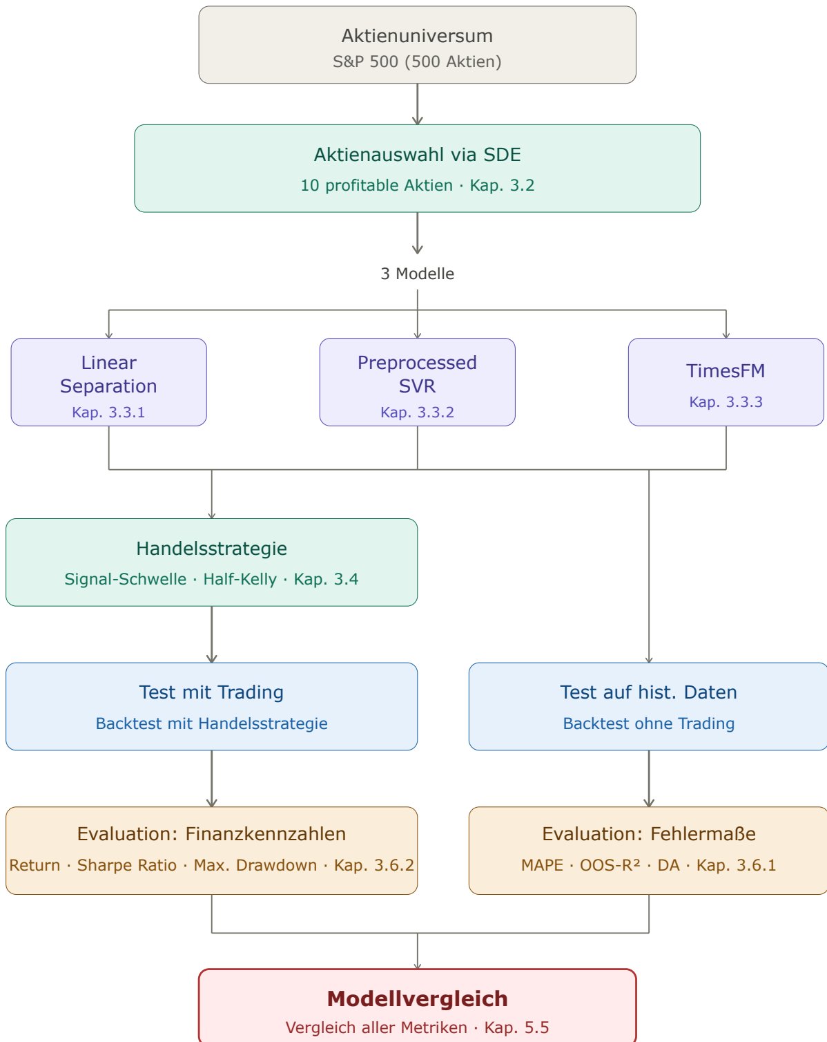
Abbildung 3.1.: Struktur der Konzeption
