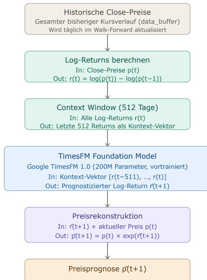
Abbildung 4.5.: TimesFM: Datenfluss der Vorhersage von neuen Kursen
