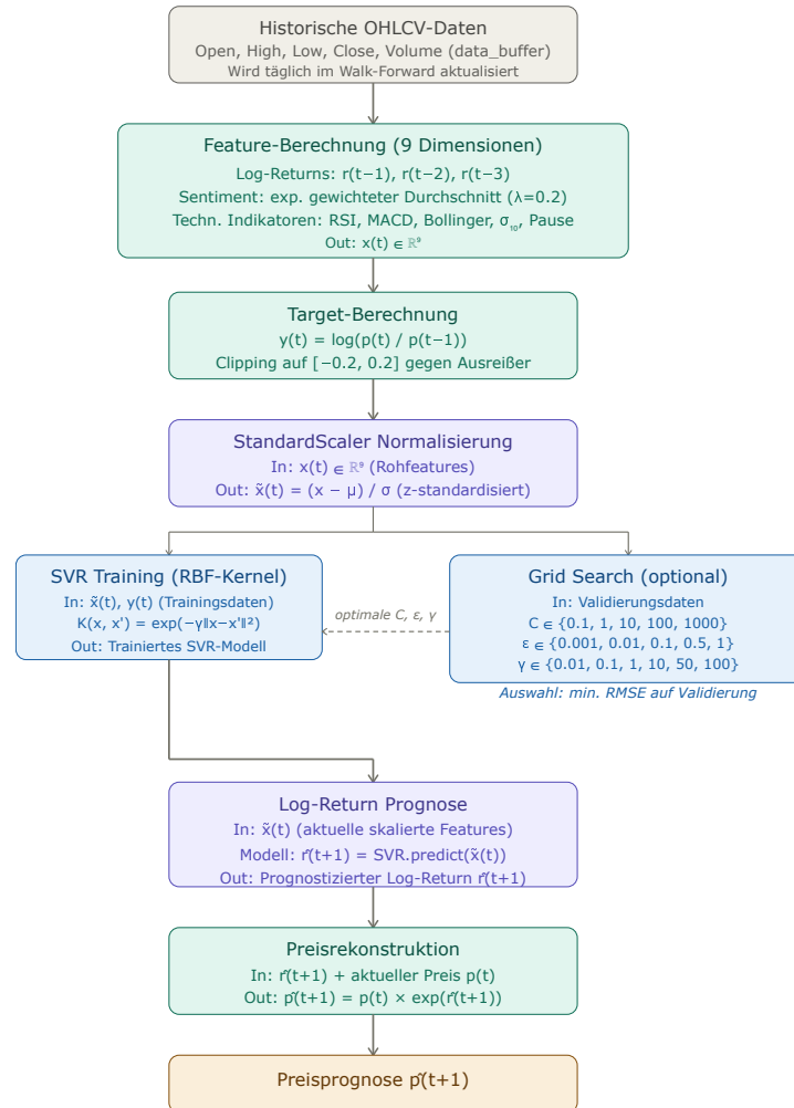
Abbildung 4.4.: Preprocessed SVR: Datenfluss von den Trainingsdaten bis zur Preisprognose
