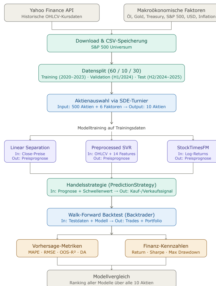
Figure 4.1.: Gesamtüberblick: Datenfluss von der Beschaffung bis zur Evaluation
