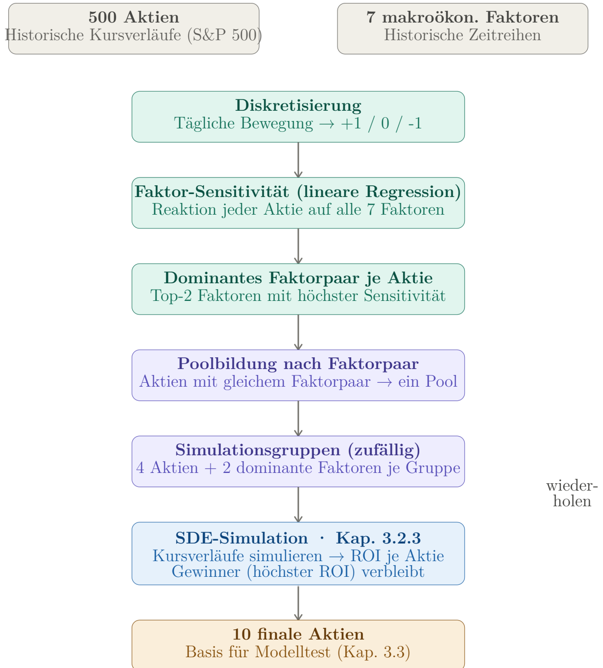
Abbildung 3.2.: Ablauf Aktienauswahl
