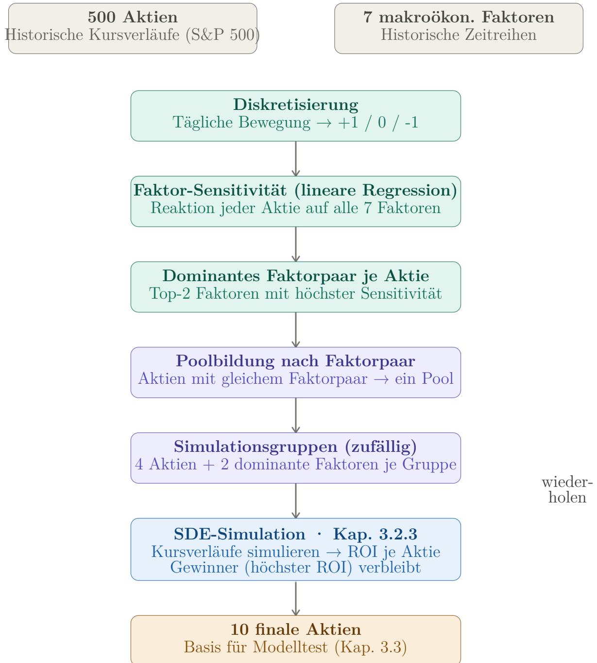
Abbildung 3.2.: Ablauf Aktienauswahl
