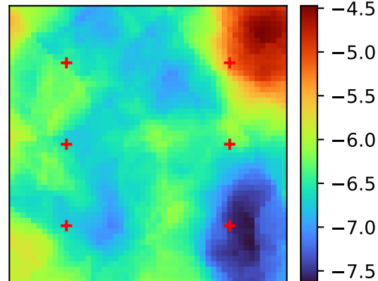
Posterior std \log_{10} K (EnKS)
