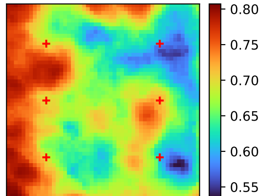
Posterior std \log_{10} K (EnKS)
