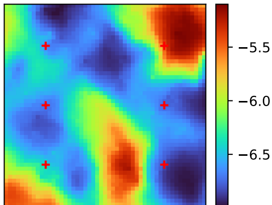
Posterior std \log_{10} K (P-Spline EnTS)
