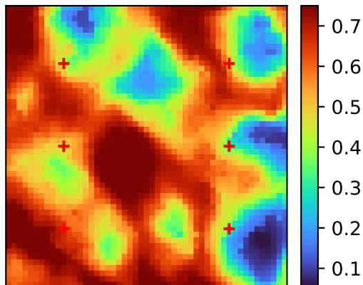
Posterior std \log_{10} K (P-Spline EnTS)
