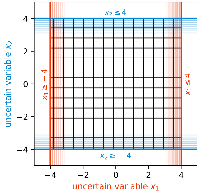
A: marginal bounds enclose a box
