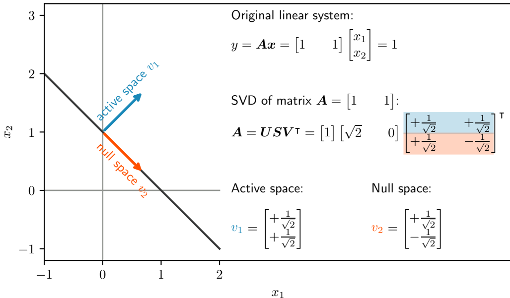
A: Linear system x_1 + x_2 = 1
