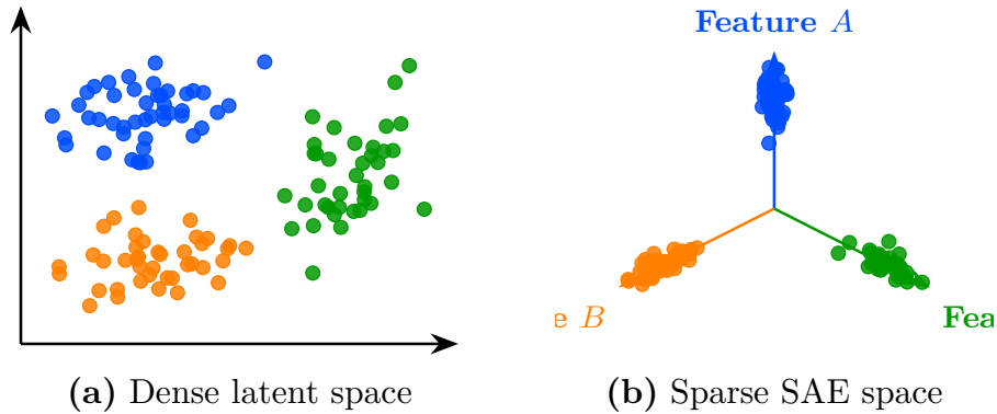
Figure 1.4: Transformation de l'espace latent dense vers une représentation sparse de type SAE. À gauche (a) , les embeddings sont entremêlés dans l'espace latent initial. À droite (b) , la représentation sparse aligne chaque concept sur un axe de feature dédié.
