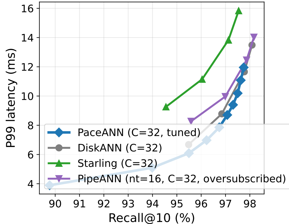
SpaceV100M
