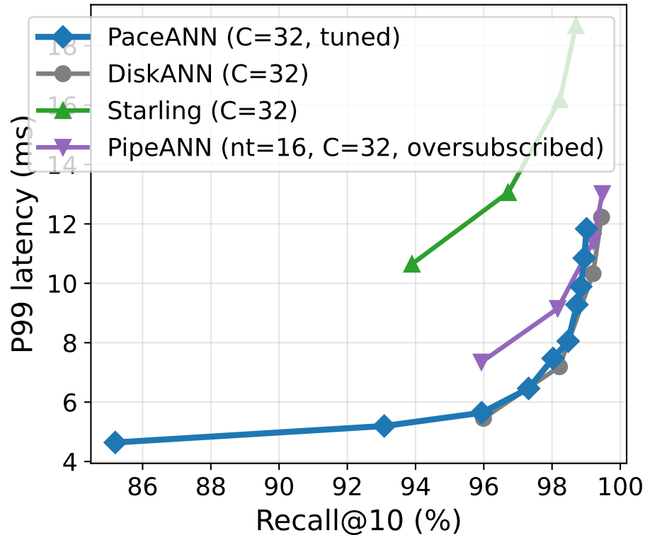
SIFT100M
