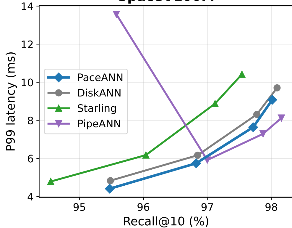
SpaceV100M
