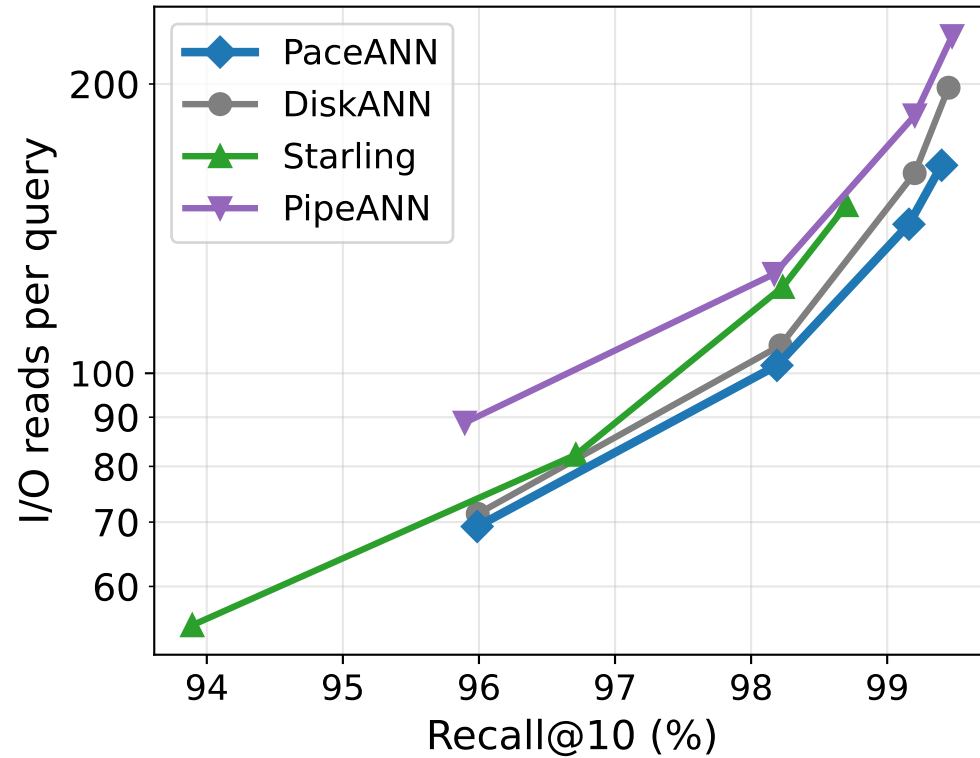
SIFT100M
