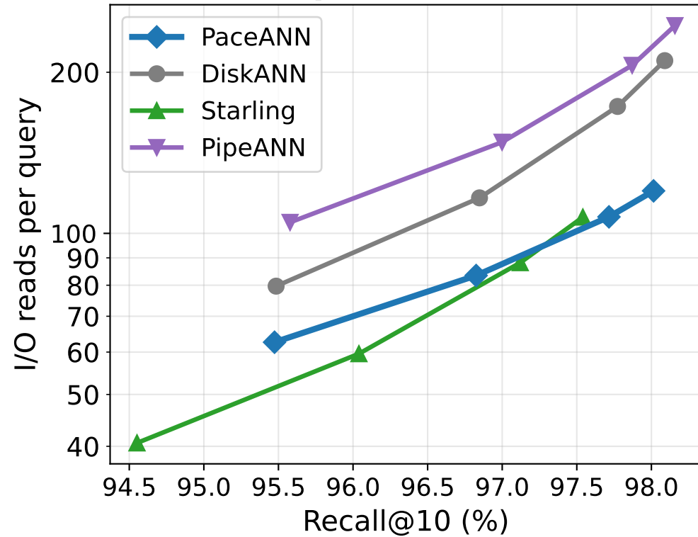
SpaceV100M
