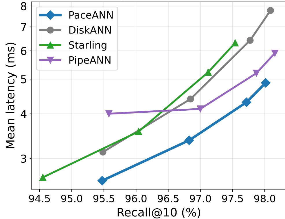
SpaceV100M
