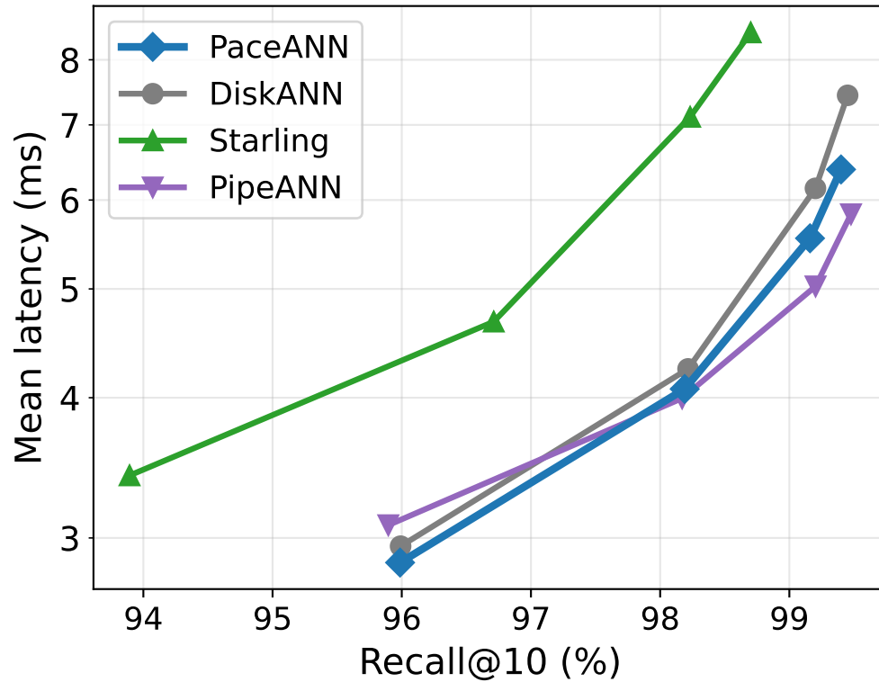
SIFT100M
