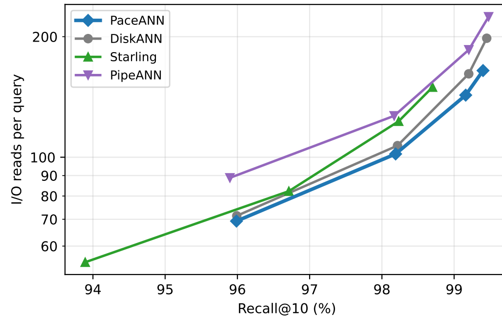
SIFT100M
