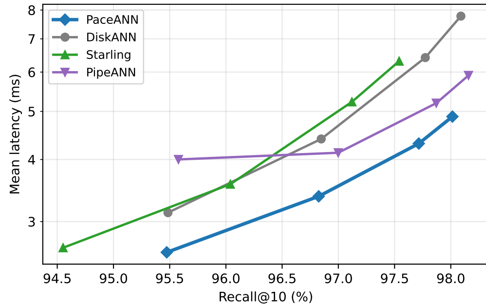
SpaceV100M
