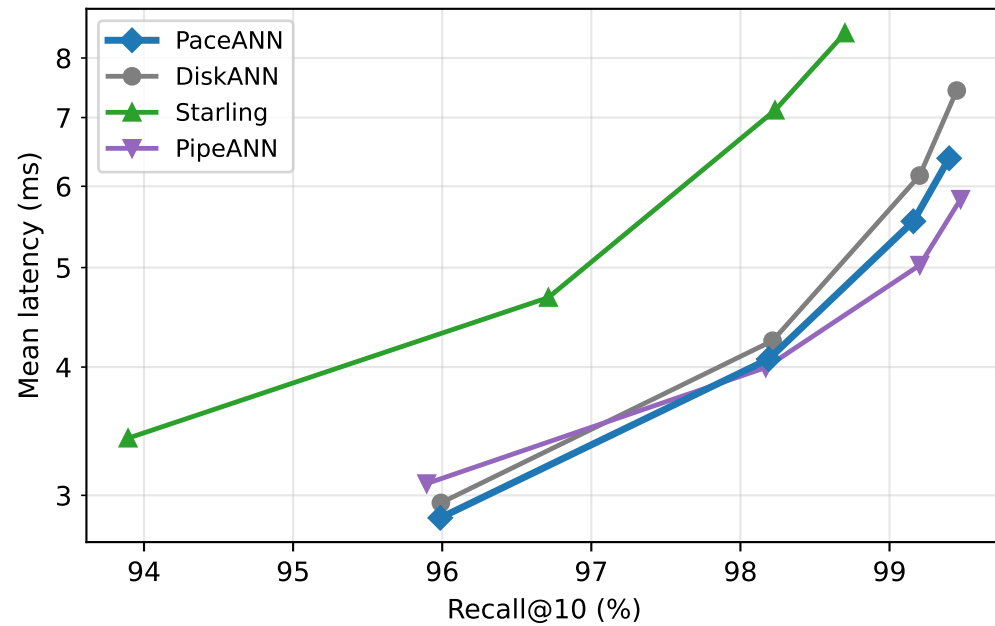
SIFT100M
