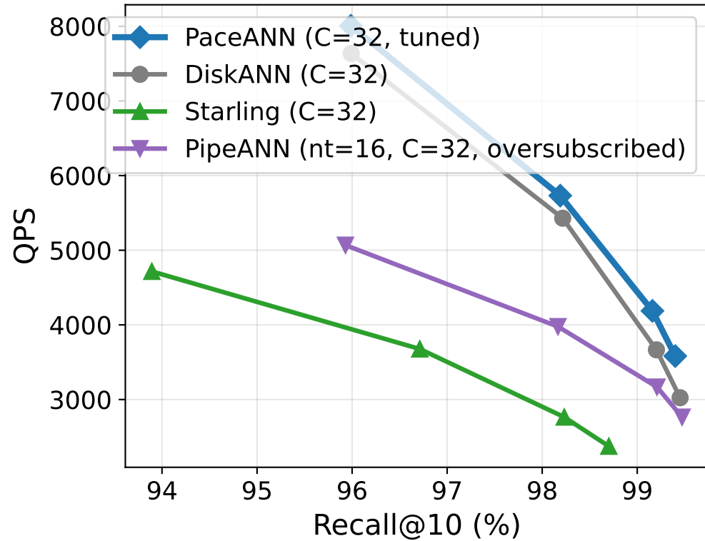
SIFT100M
