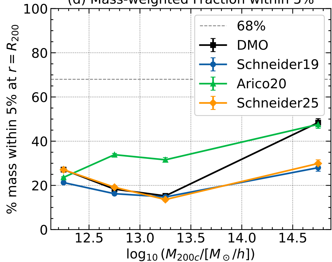
(d) Mass-weighted Fraction within 5%
