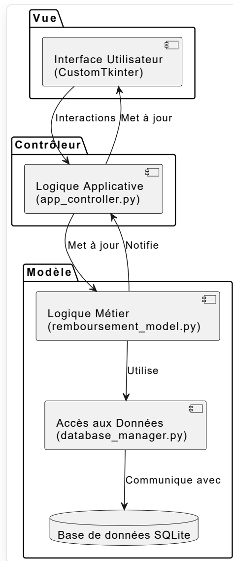
Figure 2 : Schéma d'architecture de l'application "Gestion des Remboursements"
