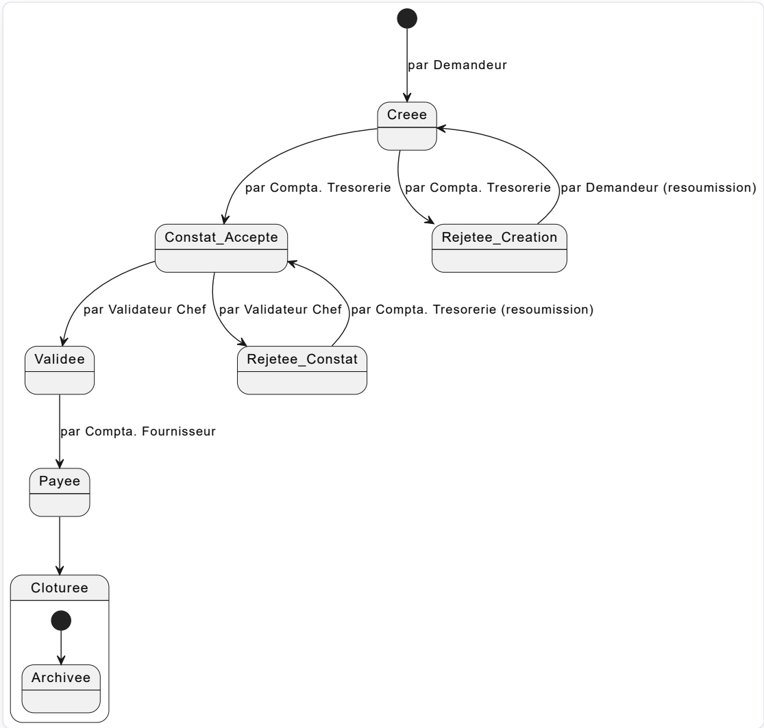
Figure 3 : Diagramme du workflow de validation des remboursements
