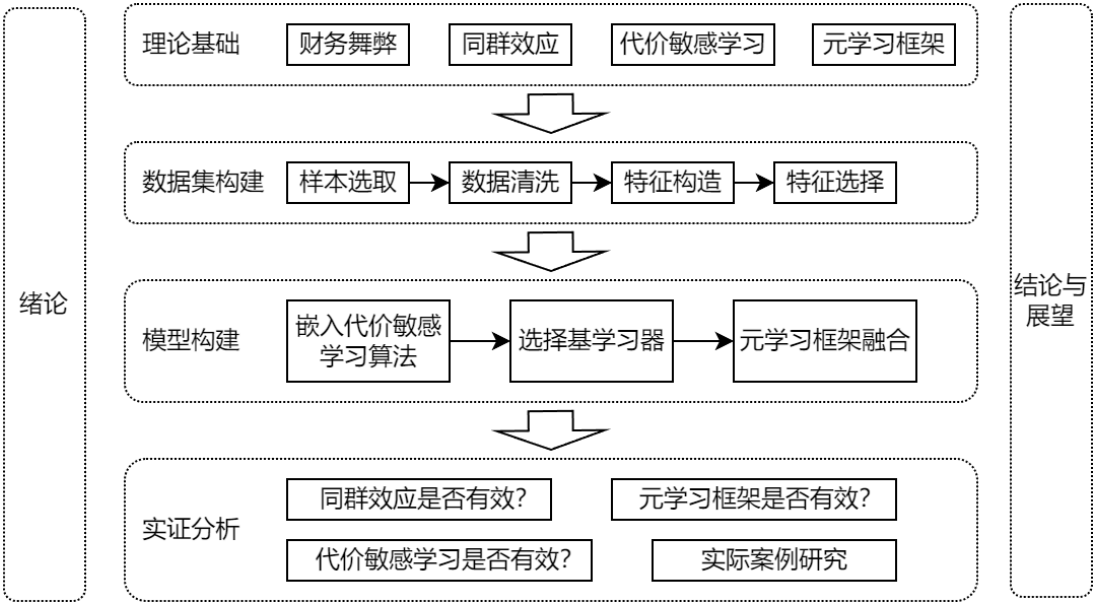
图 2.1 论文流程图
