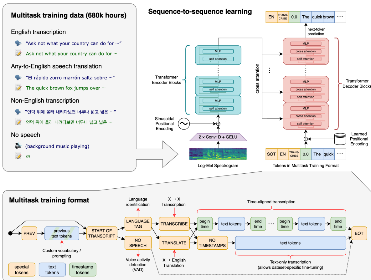
Diagrama de bloques del modelo Whisper
