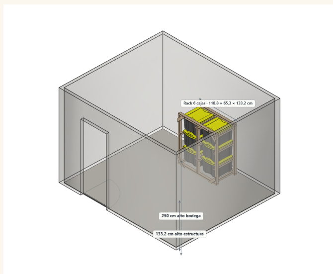
VISTA DESDE LA ENTRADA
