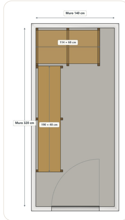
PLANTA Y MEDIDAS
