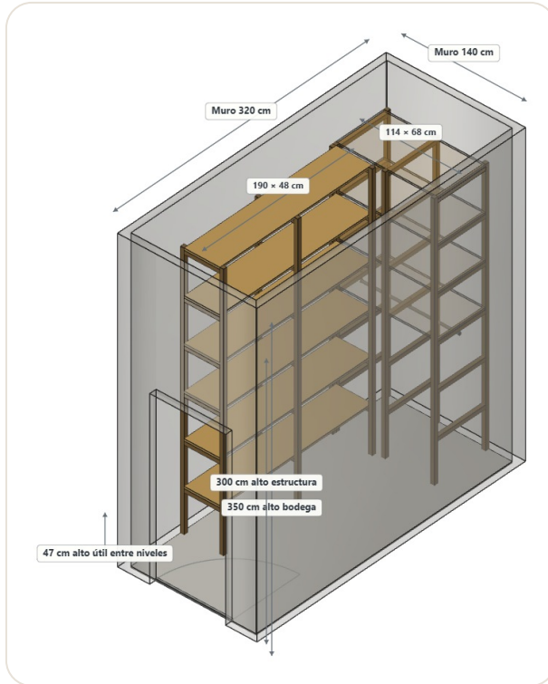
VISTA ISOMÉTRICA
